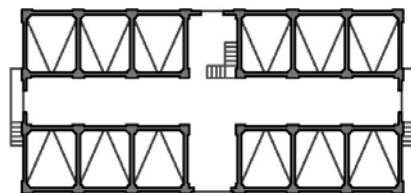
TPO H: PLANTA BAJA
