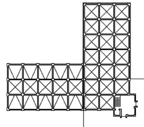
Opción B-7500 ton Option B-7500
