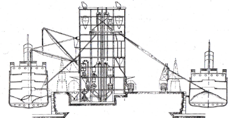
Silo de Málaga.—Sección por la torre de máquinas
