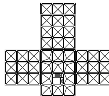
Option A-4 Opción A-4 3950 ton
